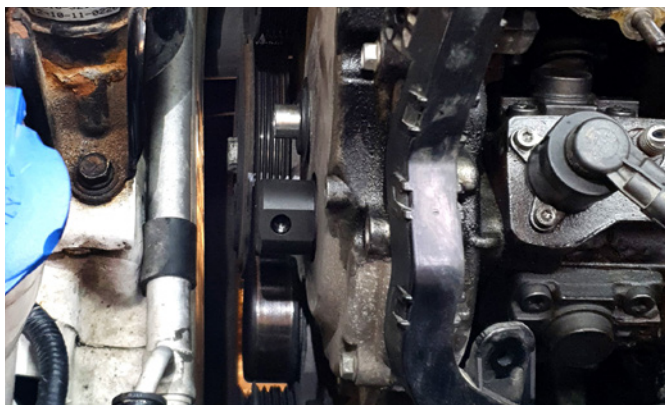
ABZIEHER FÜR HOCHDRUCKPUMPEN-KETTENRAD
